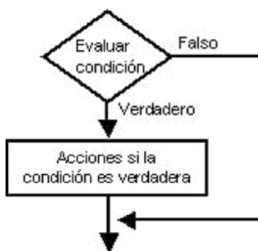
Figura 1.3: Estructura Si-Entonces
