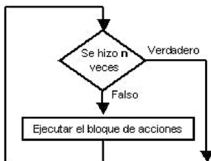
Figura 1.4: Estructura repetitiva
